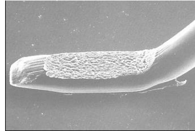
Wedge bond
